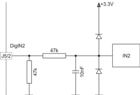
图 3-9 DigIN2 的连接
