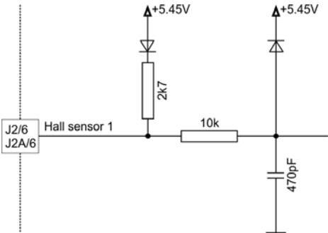
图 3-6 霍尔传感器输入端的连接（霍尔传感器 2 和 3 的连接方式类似）
