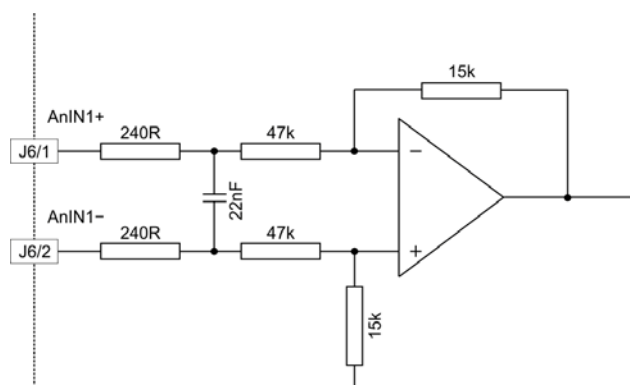
图 3-14 AnIN1 的连接 (AnIN2 的连接方式类似)
