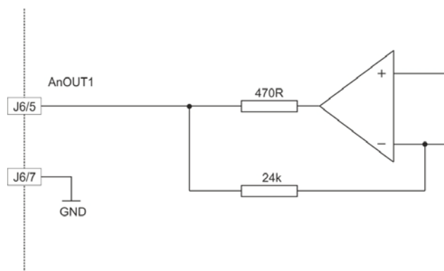
图 3-15 AnOUT1 的连接 (AnOUT2 的连接方式类似)
