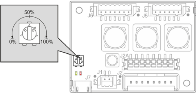
图 3-20 电位器 P1 – 安装位置和调节范围
