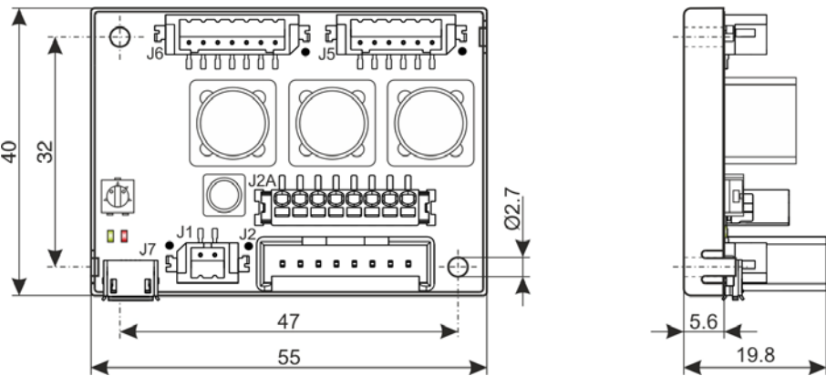
图 2-2 尺寸图 [mm]
