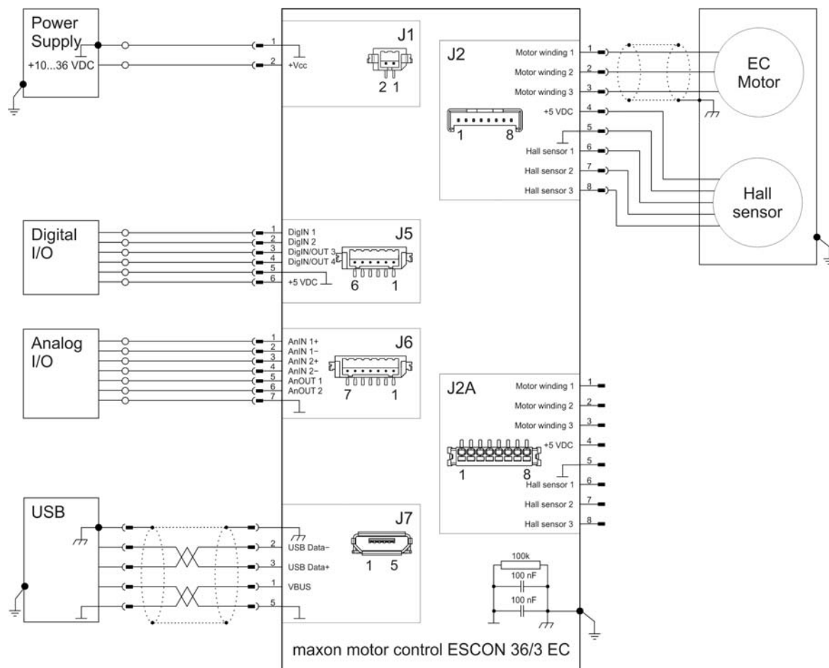
图 4-23 带霍尔传感器的 maxon EC 电机 (J2)
